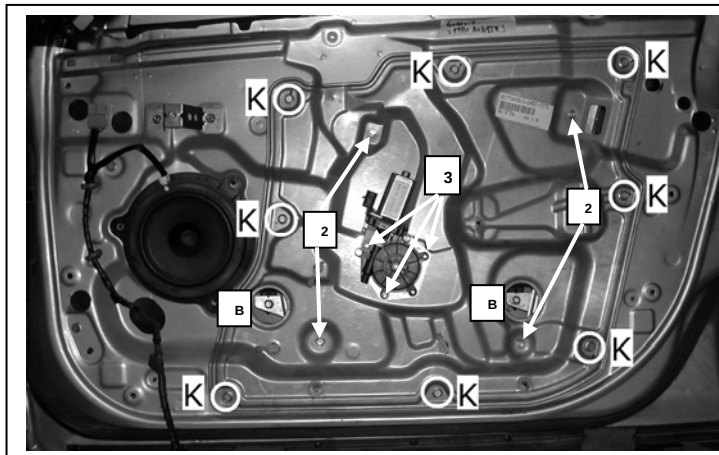
Puerta lado derecho, Portière avant droite, Right front door, Porta frente dirietta
