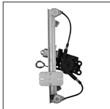
Nuestro elevavinas – notre lève-vitre – our window regulator – nosso levantador de vidro
