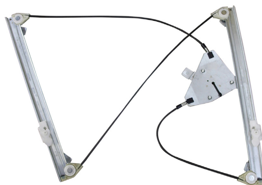
Nuestro Elevallunas / Our window regulator / Notre lève-vitre / Nosso elevador de vidro
