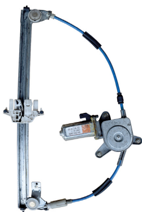
Elevallunas original / OEM window regulator / Lève-vitre original / Elevador de vidro original
