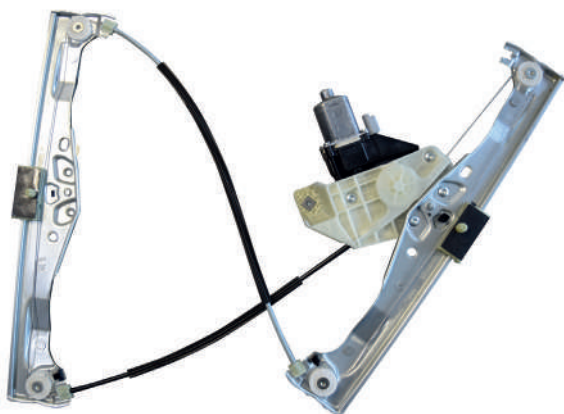
Elevallunas original / OEM window regulator / Lève-vitre original / Elevador de vidro original
