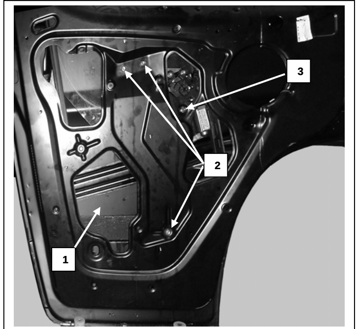
Puerta lado izquierdo, Portière arrière gauche, Left rear door, Porta traseira esquerda
