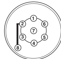
Tikobling av ledninger i den 7-polete kontakten
