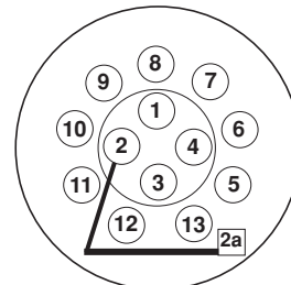
Tikobling av ledninger i den 13-poete kontakten
