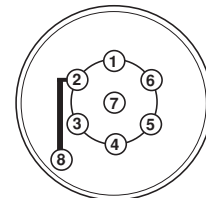
Tikobling av ledninger i den 7-poete kontakten
