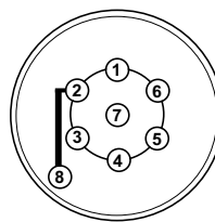
Tilkobling av ledninger i den 7-polete kontakten
