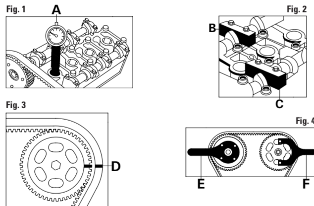
FIGURA 1 Inserire l'apposito attrezzo di comparazione A, sul cilindro N° 1. FIGURA 2 Smontare il cappelotto: del 2° cilindro lato scarico dell'albero a camme (per modello JTS); del 2° cilindro lato aspirazione dell'albero a camme (per modello Delta); del 3° cilindro lato aspirazione dell'albero a camme (per tutti i modelli); del 3° cilindro lato scarico dell'albero a camme (per modello Delta); del 4° cilindro lato scarico dell'albero a camme (per modello Barchetta); ed inserire gli appositi attrezzi bloccaggio B e C. FIGURA 3 Controllare il corretto allineamento delle tacche di fase D. FIGURA 4 Attrezzi per il mantenimento della tensione dell'albero a camme E ed F.
