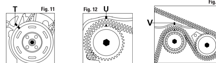
FIGURA 11 Controllare il corretto allineamento delle tacche di fase T. FIGURA 12 Controllare il corretto allineamento delle tacche di fase U. FIGURA 13 Controllare il corretto allineamento delle tacche di fase V.
