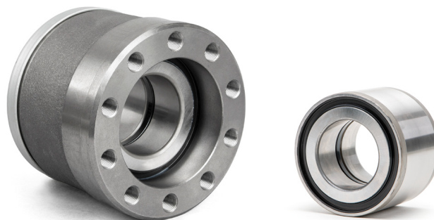
Foto 1: Moduł osi FAG (TAM) – nr części: 632203.H195 (po lewej), Moduł piasty FAG (THU) – nr części: 201050 (po prawej)
