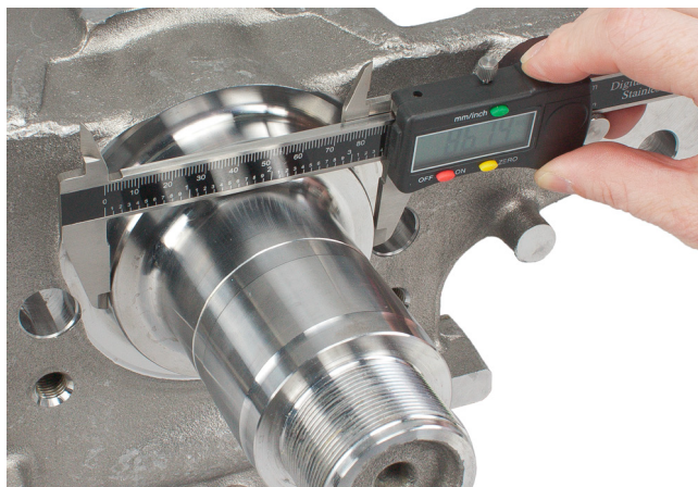
Foto 2: Aby określić, który z trzech pierścieni ochronnych należy zamontować, należy zmierzyć średnicę gniazda uszczelniającego
