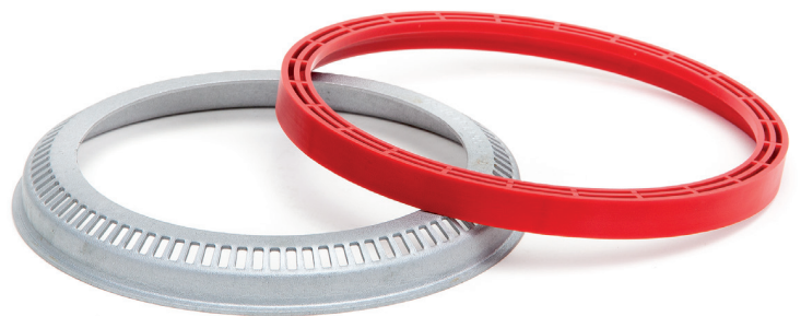
Bague de capteur ABS réf. 434 0497 10 avec outillage spécial pour la pose
