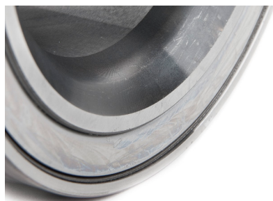
Figura 3: Ansamblul butucului de camion cu muchie teșită
