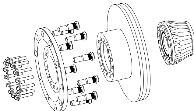
Figura 1: În cazul punților marcate cu ID-ul S63U, pe lângă modulul rulmentului de roată, trebuie să se înlocuiască și discul de frână, dispozitivul de fixare a roții, prezoanele roților și șuruburile de fixare.
