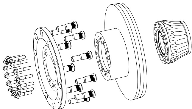
Obrázek 1: U náprav s identifikátorem S63U se musí vedle modulu ložiska kola předavně vyměnit také brzdový kotouč, uchycení kola, šrouby kola a upevňovací šrouby
