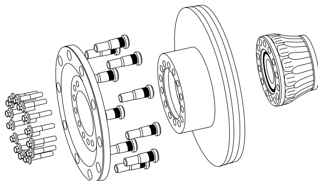
Kuva 1: Akseleissa, joiden tunniste on S63U, on pyöränlaakerimoduulin lisäksi vaihdettava myös jarrulevy, pyörän kiinnitin, pyöränpultit ja kiinnitysruuvit
