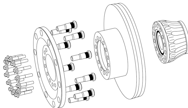
Foto 1: W osiach oznaczonych symbolem S63U, oprócz modułu osi FAG trzeba wymienić również: tarczę hamulcową, pierścień nośny, szpilki koła i nowe śruby.
