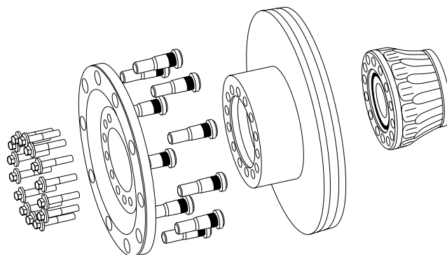
Рисунок 1: Для осей, маркированных номером S63U, в дополнение к ступичному модулю, должны заменяться тормозной диск, крепление колеса, резьбовые шпильки и гайки
