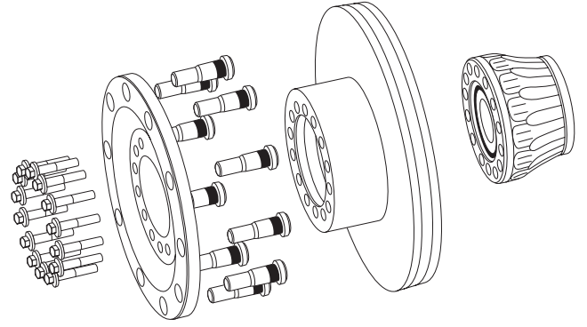
Resim 1: S63U nolu akslarda tekerlek rulmanı modülüne ek olarak fren diski, tekerlek, tekerlek saplaması ve sabitleme vidaları da ayrıca değiştirilmelidir.
