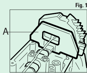
FIGURA 1: Inserire l'apposito attrezzo di bloccaggio degli alberi a camme A.
