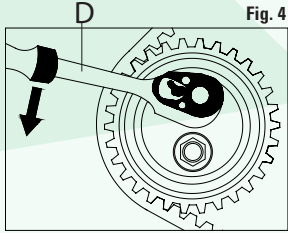
FIGURA 2: Allentare il bullone di bloccaggio del tendicinghia della distribuzione. FIGURA 3-4: Inserire l'apposito attrezzo di misurazione della tensione C, nel punto indicato, e ruotare il tendicinghia in senso antiorario fino al raggiungimento del valore di 45 SKT. FIGURA 5: Inserire l'apposito attrezzo N°11 5 060. Agendo sul tendicinghia, portare l'indicatore mobile fino alla corretta tensione; serrare quindi i bulloni di bloccaggio.
