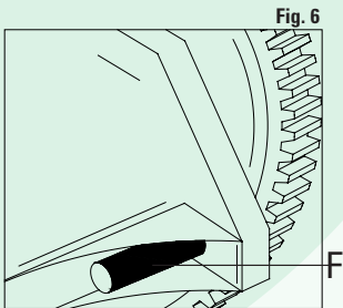
FIGURA 6: Inserire l'apposito attrezzo di bloccaggio dell'albero motore F, N°11 2 300 .
