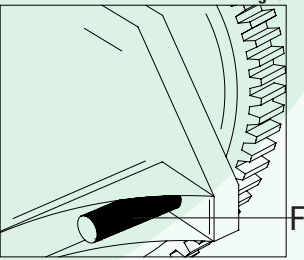
FIGURA 6: Insertar la herramienta especial para inmovilización de cigüeñal motor F, N°11 2 300 .
