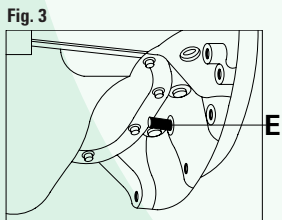
FIGURA 3 Insertar la herramienta de inmovilización del volante motor E. FIGURA 4 Girar el cigüeñal hasta alinear el orificio para la puesta en fase del motor y proceder a instalar la herramienta especial de inmovilización F.
