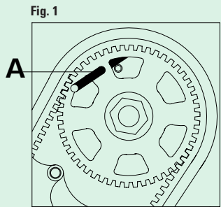
FIGURA 1 Inserire l'apposito attrezzo di bloccaggio dell'albero a camme A.
