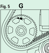
FIGURA 5 Insertar la herramienta específica para inmovilizar la polea de la bomba de inyección G.
