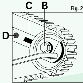
FIGURA 2 Aflojar el tornillo de fijación B, girar el tensor de correa en sentido contrario a las agujas del reloj, alinear el indicador C en el centro de la zona de control D. Luego proceda apretar el tornillo de fijación B.
