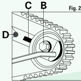
FIGURA 2 Allentare il bullone di bloccaggio B e ruotare il tendicinghia in senso antiorario; allineare l'indicatore C al centro della zona di controllo D e serrare, quindi, il bullone di bloccaggio B.
