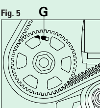
FIGURA 5 Inserire l'apposito attrezzo di bloccaggio della pompa di iniezione G.
