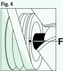
FIGURA 4 Controllare il corretto allineamento della tacca di fase F. FIGURA 5 Controllare il corretto allineamento della tacca di fase G.
