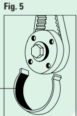
FIGURA 4 Inserire l'apposito attrezzo di bloccaggio del volano G. FIGURA 5 Inserire l'apposito attrezzo di bloccaggio della cinghia di distribuzione H. FIGURA 6 Controllare il corretto allineamento delle tacche di fase I.
