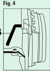
FIGURA 4 Insertar la herramienta de inmovilización del volante motor G. FIGURA 5 Insertar la herramienta específica para inmovilizar la correa de distribución H. FIGURA 6 Verificar la correcta alineación de las marcas de puesta en fase I.
