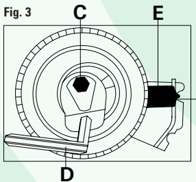
FIGURA 3 Allentare il bullone di bloccaggio, C, e ruotare il tendicinghia in senso antiorario tramite la chiave esagonale D, quindi, allineare l'indicatore, E, al centro della zona di controllo, F, serrare quindi il bullone di bloccaggio C.
