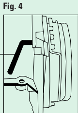
FIGURA 4 Inserire l'apposito attrezzo di bloccaggio del volano G. FIGURA 5 Inserire l'apposito attrezzo di bloccaggio della cinghia di distribuzione H. FIGURA 6 Controllare il corretto allineamento delle tacche di fase I.
