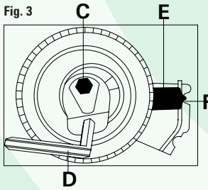
FIGURA 3 Aflojar el tornillo de fijación C. Girar el tensor de la correa en sentido contrario a las agujas del reloj utilizando para ello la llave hexagonal D. Alinear el indicador E con el centro de la zona de control F. Por último, apretar el tornillo de fijación C.
