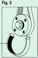
FIGURA 4 Insertar la herramienta de inmovilización del volante motor G. FIGURA 5 Insertar la herramienta específica para inmovilizar la correa de distribución H. FIGURA 6 Verificar la correcta alineación de las marcas de puesta en fase I.
