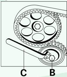
FIGURA 2 Allentare il bullone di bloccaggio B e ruotare in senso orario il tendicinghia utilizzando la chiave C agendo sull'eccentrico di registro.
