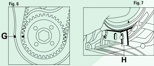
FIGURA 6 Controllare il corretto allineamento delle tacche di fase G. FIGURA 7 Inserire l'apposito attrezzo di bloccaggio del volano H.
