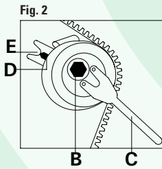
FIGURA 2 Aflojar el tornillo de fijación B, girar el tensor de correa utilizando la herramienta especial C primero hacia la izquierda y luego hacia la derecha hasta que el indicador D se encuentre en la posición E. Luego, vuelva apretar el tornillo de fijación B.
