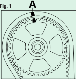
FIGURA 1 Controllare il corretto allineamento della tacca di fase A.
