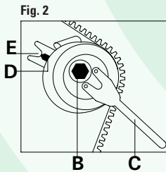
FIGURA 2 Allentare il bullone di bloccaggio B e ruotare il tendicinghia tramite l'apposito attrezzo di tensionamento C, prima in senso antiorario e poi in senso orario fino a quando l'indicatore D si trovi nella posizione E; serrare quindi il bullone di bloccaggio B.
