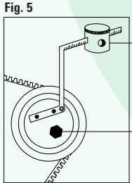
FIGURA 5 Aflojar el tornillo de fijación E. Insertar la herramienta específica para tensado de correas con su peso relativo. (F:100 mm para motores 16V; (F:140 mm para motores VR). Verificar que el brazo de la herramienta permanezca en posición horizontal. Por último, apriete el tornillo de fijación E.
