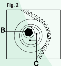
FIGURA 2 Allentare il bullone di bloccaggio B e ruotare in senso antiorario il tendicinghia sull'eccentrico di registro C fino alla corretta tensione; serrare quindi il bullone di bloccaggio B. FIGURA 3 Inserire l'apposito attrezzo di misura del tensionamento D, nel punto indicato, ed agire sul tendicinghia fino al valore di 30 unità SEEM.
