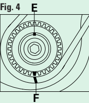
FIGURA 4 Verificar la correcta alineación de las marcas de puesta en fase E y F.
