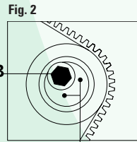
FIGURA 2 Aflojar el tornillo de fijación B, girar el tensor de correa sobre el excéntrico de regulación C en sentido contrario a las agujas de reloj hasta lograr la tensión correcta. Luego vuelva apretar el tornillo de fijación B.
