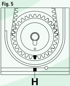
FIGURA 4 Insertar la herramienta de inmovilización del volante motor G. FIGURA 5 Verificar la correcta alineación de las marcas de puesta en fase H.
