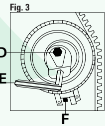
FIGURA 2 Controllare il corretto allineamento delle tacche di fase B e C. FIGURA 3 Allentare il bullone di bloccaggio D e ruotare in senso antiorario il tendicinghia, utilizzando la chiave esagonale E sull'eccentrico di registro; allineare l'indicatore F nella zona di controllo e serrare, quindi, il bullone di bloccaggio D.
