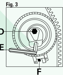
FIGURA 2 Verificar la correcta alineación de las marcas de puesta en fase B y C. FIGURA 3 Aflojar el tornillo de fijación D. Girar el tensor de la correa en sentido contrario a las agujas del reloj, actuando con la llave E sobre el excéntrico de regulación hasta lograr alinear el indicador F dentro de la zona de control. Por ultimo, apretar el tornillo de fijación D.
