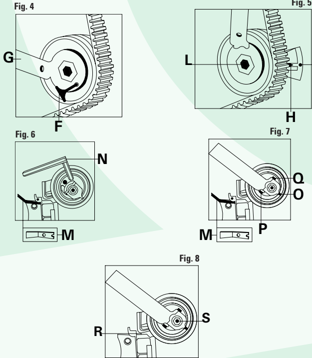
FIGURA 4 Insertar la herramienta especial para inmovilización del tensor de correa F. Girar en sentido contrario a las agujas del reloj manteniendo en tensión el tensor de correa utilizando la herramienta G. FIGURA 5 Después de retirar la herramienta de inmovilización, girar el tensor de correa en sentido de las agujas del reloj y alinear el indicador H al centro de la zona de control I. Por ultimo, apretar el tornillo de fijación L. FIGURA 6 Insertar la herramienta especial para inmovilización del tensor de correa M. Girar en sentido contrario a las agujas del reloj manteniendo en tensión el tensor de correa utilizando la llave hexagonal N. FIGURA 7 Girar el tensor de correa en sentido de las agujas del reloj hasta lograr alinear las marcas O y P. Girar el tensor de correa en sentido contrario al de las agujas del reloj hasta lograr alinear las marcas de alineación Q y Q. Por ultimo, extraer la herramienta de inmovilización M. FIGURA 8 Girar el tensor de correa en sentido de las agujas del reloj hasta llevar el juego de regulación R hasta un valor de 4 mm. Luego apretar el tornillo S. FIGURE 4 Introduire l'outil approprié de blocage du tendeur de courroie F, tourner dans le sens contraire aux aiguilles de la montre le tendeur de courroie en utilisant l'outil G. FIGURE 5 Après avoir extrait l'outil de blocage, tourner le tendeur de courroie dans le sens des aiguilles de la montre, aligner l'indicateur H au centre de la zone de contrôle I, serrer ensuite le boulon de blocage L. FIGURE 6 Introduire l'outil approprié de blocage du tendeur de courroie M, tourner le tendeur de courroie dans le sens contraire aux aiguilles de la montre en utilisant la clef hexagonale N. FIGURE 7 Tourner le tendeur de courroie dans le sens des aiguilles de la montre jusqu'à aligner les points de repère O et P. Tourner dans le sens contraire aux aiguilles de la montre le tendeur de courroie jusqu'à aligner les points de repère Q et Q, extraire l'outil de blocage M. FIGURE 8 Tourner le tendeur de courroie dans le sens des aiguilles de la montre jusqu'à régler le jeu R à la valeur de 4mm, serrer ensuite le boulon S.
