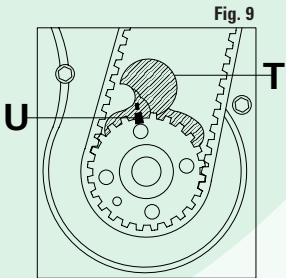
FIGURA 9 La marca de fase en la herramienta inmovilizadora T debe estar en línea con la marca de fase del cigüeñal U.
