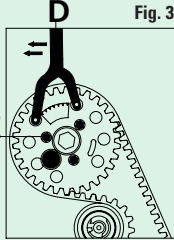
FIGURA 1 Inserire l'apposito attrezzo di bloccaggio dell'albero a camme A. FIGURA 2 Controllare il corretto allineamento della tacca di fasatura verificando che essa sia allineata con l'intaglio sul mozzo del pignone dell'albero a camme: B per motori 4 cilindri e C per motori 3 cilindri. FIGURA 3 Inserire l'apposito attrezzo D, per mantenere gli ingranaggi in tensione e serrare le 3 viti E, sfalsate di 120° l'una dall'altra.
