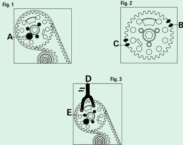
FIGURA 1 Insertar la herramienta especial de inmovilización de árbol de levas A. FIGURA 2 Verificar que la marca de puesta a tiempo este correctamente alineada con la muesca tallada sobre el mozo del piñón del árbol de levas; B para motores 4 cilindros y C para motores 3 cilindros. FIGURA 3 Insertar la herramienta especial D para mantener la correa en tensión entre los engranajes, y apretar los 3 tornillos E, los cuales están distanciados 120° entre sí.
