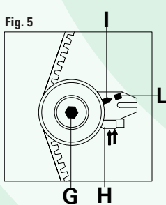
FIGURA 5 Allentare il bullone di bloccaggio G e, spingendo nel punto indicato H, quindi, portare l'indicatore mobile I nella posizione di massima tensione e, dopo aver fatto coincidere il punto I con il Punto L, serrare il bullone di bloccaggio G.
