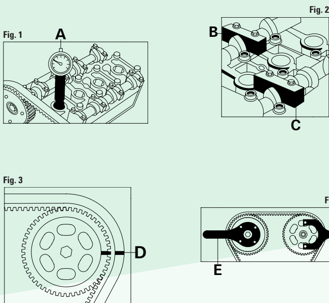
FIGURA 1 Inserire l'apposito attrezzo di comparazione A, sul cilindro N° 1. FIGURA 2 Smontare il cappellotto: del 2° cilindro lato scarico dell'albero a camme (per modelli: Lancia Lybra, Coupè, Bravo e Marea); del 3° cilindro lato scarico dell'albero a camme (per modello Lancia K); del 4° cilindro lato aspirazione dell'albero a camme (per modelli: Lancia K, Lybra, Coupè, Bravo e Marea). FIGURA 3 Controllare il corretto allineamento delle tacche di fase D. FIGURA 4 Attrezzi per il mantenimento della tensione dell'albero a camme E ed F.
