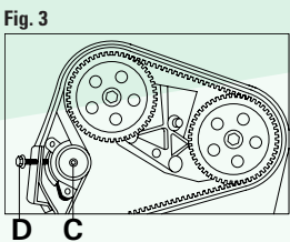
FIGURA 3 Aflojar el tornillo de fijación C. Insertar la herramienta específica D para tensado de correa, atomillándola hasta obtener la tensión correcta. Por último, apretar el tornillo de fijación C.
