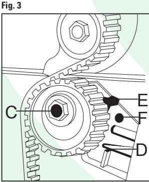
FIGURA. 3 Aflojar el tornillo de fijación C. Actuando en el punto indicado D del tensor automático, llevar al indicador móvil E hasta la posición de máxima tensión, y luego de haber hecho coincidir el punto E con el punto F, apretar el tornillo de fijación C. FIGURE 3 Desserer le boulon de blocage C, en intervenant au point indiqué D du tendeur automatique, placer l'indicateur mobile E dans la position majeure tension, et après avoir fait coïncider le point E avec le point F, serrer le boulon de blocage C.
