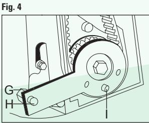
FIGURA 4 Smontare il bullone della pompa dell'olio G e installare al suo posto il prigioniero dell'attrezzo di bloccaggio H. Ruotare l'albero motore fino al PMS del cilindro N° 1 e verificare il corretto posizionamento del grano della puleggia dell'albero motore L.
