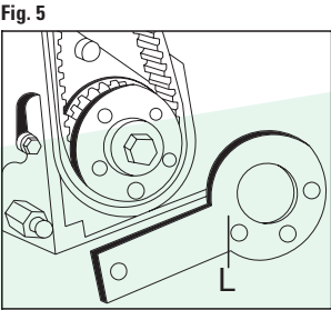
FIGURA. 4 Desmontar el tornillo de la bomba de aceite G, y en su lugar, instalar el prisionero de la herramienta de inmovilización H. Rotar el cigüeñal hasta alcanzar el PMS del cilindro N° 1 y verificar la correcta posición de la marca de la polea del cigüeñal L. FIGURA. 5 Insertar la herramienta especial de inmovilización del cigüeñal L.
