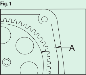
FIGURA 1: Controllare il corretto allineamento delle tacche di fase A. FIGURA 2: Controllare il corretto allineamento delle tacche di fase B.
