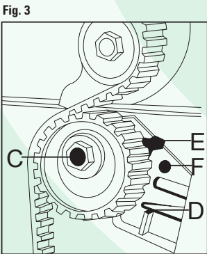
FIGURA 3 Allentare il bullone di bloccaggio C, agendo nel punto indicato, D, del tenditore automatico; portare l'indicatore mobile, E, nella posizione di massima tensione, e, dopo aver fatto coincidere il punto E con il Punto F, serrare il bullone di bloccaggio C. FIGURE 3 Unloose blocking bolt C, operating on indicated point D of the automatic tensioner, move mobile indicator E at the maximum tension position and tighten blocking bolt C after having aligned point E with point F.
