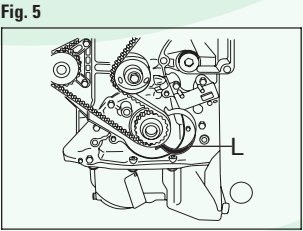
FIGURA 3 Insertar la herramienta para inmovilización de polea de cigüeñal motor H. FIGURA 4 Insertar la herramienta de inmovilización del volante motor I. FIGURA 5 Herramienta inmovilizadora de correa de distribución L.
