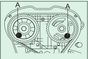
FIGURA 1 Inserire l'apposito attrezzo di bloccaggio dell'albero a camme A.
