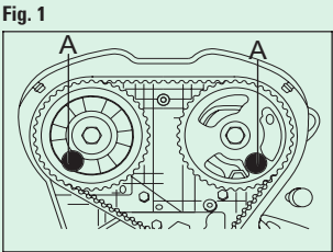
FIGURA 1 Insertar la herramienta especial de inmovilización de árbol de levas A.
