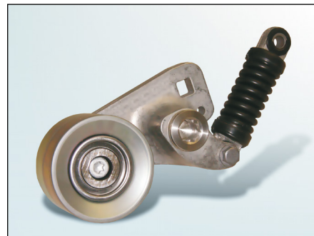
Slika 2: 534 0340 10 (aktualna izvedba)
