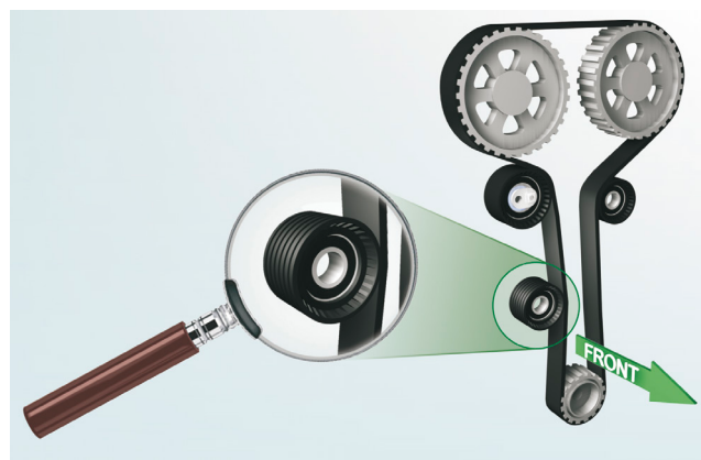
Figura 1: Cursa curelei și poziția roilor în motorul F4R
