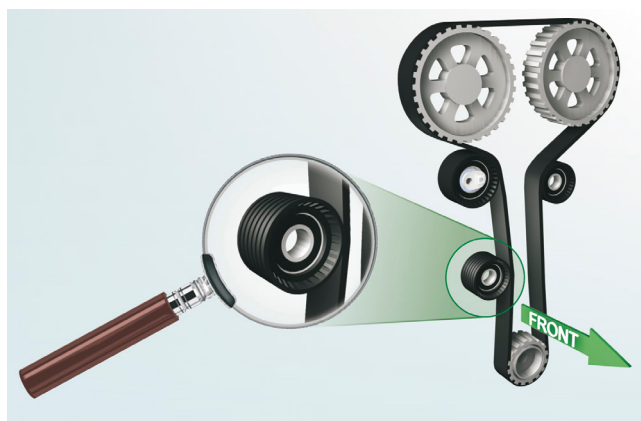
Εικόνα 1: Πορεία του ιμάντα και θέσεις τροχαλιών σε κινητήρα F4R
