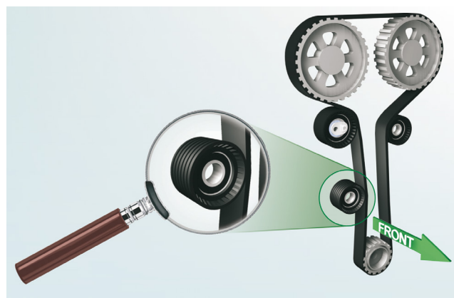
Kuva 1: F4R moottorin hihnankierto ja osien sijainti
