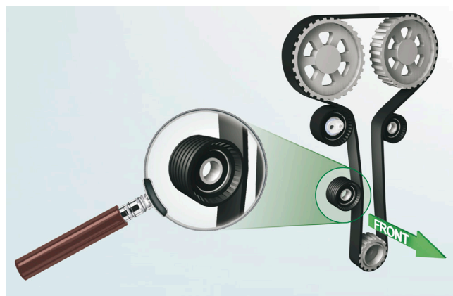
1. ábra: Szíjmenet és görgőpozíció az F4R-motorban
