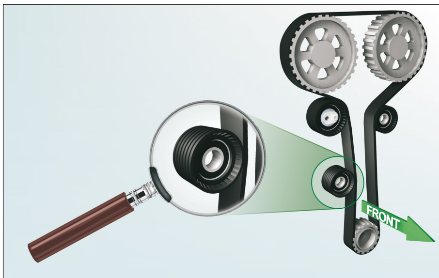
Slika 1: potek jermenov in pozicije valjev v motorju F4R
