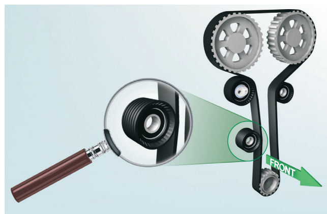
Зображення 1: Траєкторія ремня і положення роликів у двигуні F4R
