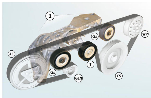
Рисунок 1: 534 0243 10 – кронштейн с натяжителем на схеме привода вспомогательных агрегатов
