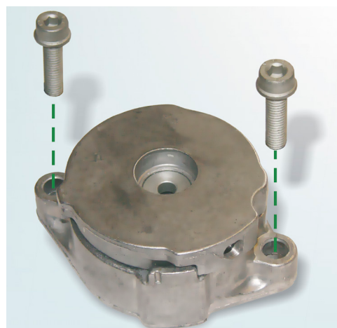
Снимка 1: Модел на INA с два болта M8x35
