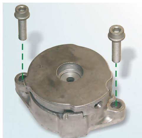
Obrázek 1: INA – provedení se dvěma šrouby M8x35
