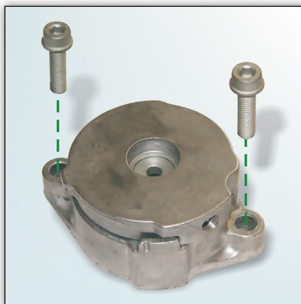
Slika 1: Izvedba INA z dvema vijakoma M8x35
