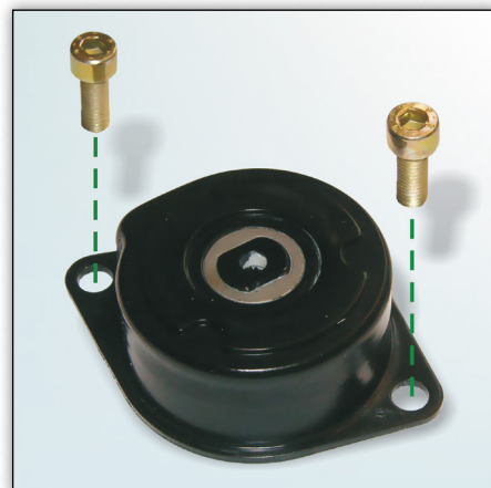
Slika 2: Izvedba z dvema vijakoma M8x22
