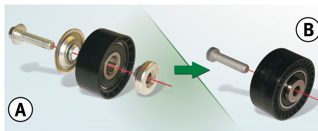
Styrerulle 532 0433 10, eksisterende specifikation (A) og ny specifikation (B)
