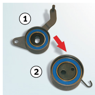
Obrázek 1: Nahrazená napínací kladka 531 0166 20 (1) a její následovník 531 0819 10 (2)
