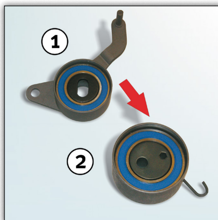
Obrázok 1: Nahradená napínacia kladka 531 0166 20 (1) a jej nasledovník 531 0819 10 (2)
