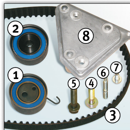
Obrázok 2: Obsah balenia 530 0492 10
