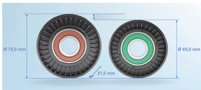
Снимка 2: Отклоняваща ролка 532 0404 30 за автомобили с бензинов двигател (ляво) и отклоняваща ролка 532 0406 30 за автомобили с дизелов двигател (дясно)
