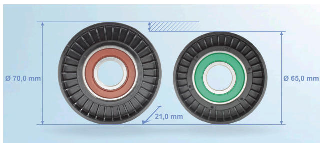
Billede 2: Afbøjningsremskive 532 0404 30 til køretøjer med en benzinmotor (venstre) og afbøjningsremskive 532 0406 30 til køretøjer med en dieselmotor (højre)
